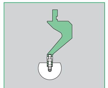
Пример монтажа с радиусной линейкой Nr. 17 R20
